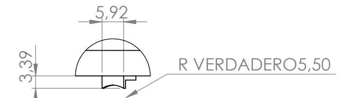
DETALLE A ESCALA 1 : 1
